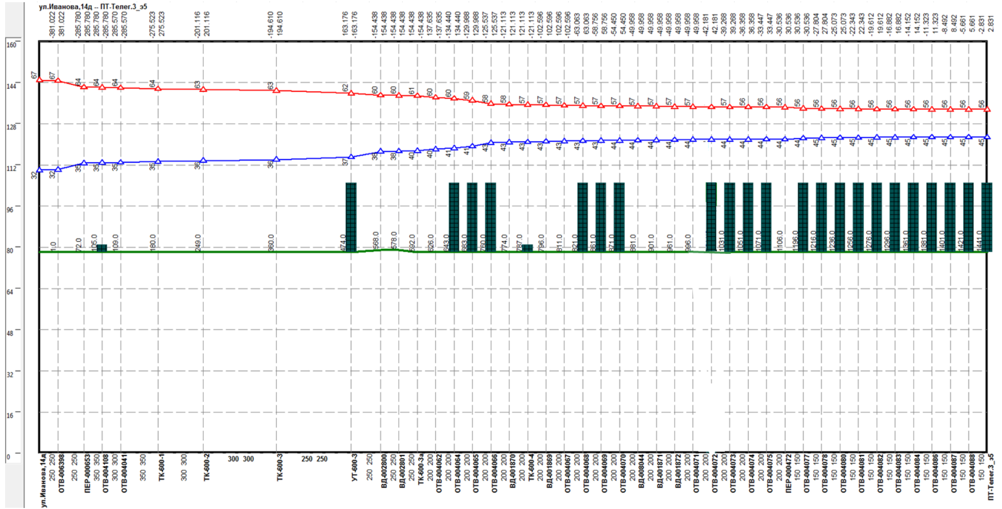
Рисунок 1.82 –Результат гидравлического расчета - график гидравлических режимов по пути теплоносителя от котельной ул. Иванова, 14б до ПТ-Телег.3_э5
