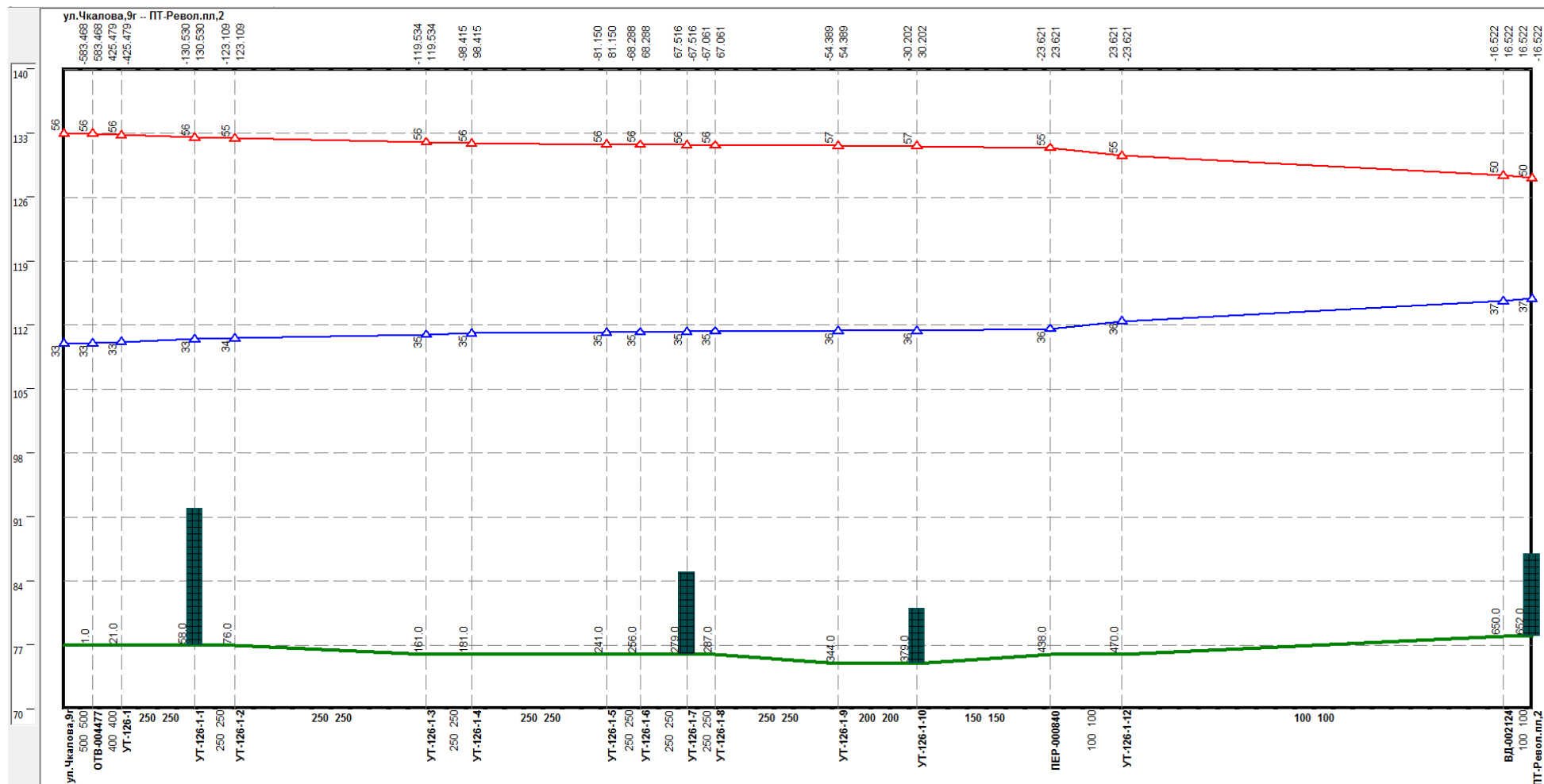
Рисунок 1.116 –Результат гидравлического расчета - график гидравлических режимов по пути теплоносителя от котельной Чкалова, 9д до ПТ-Революция, пл.2
