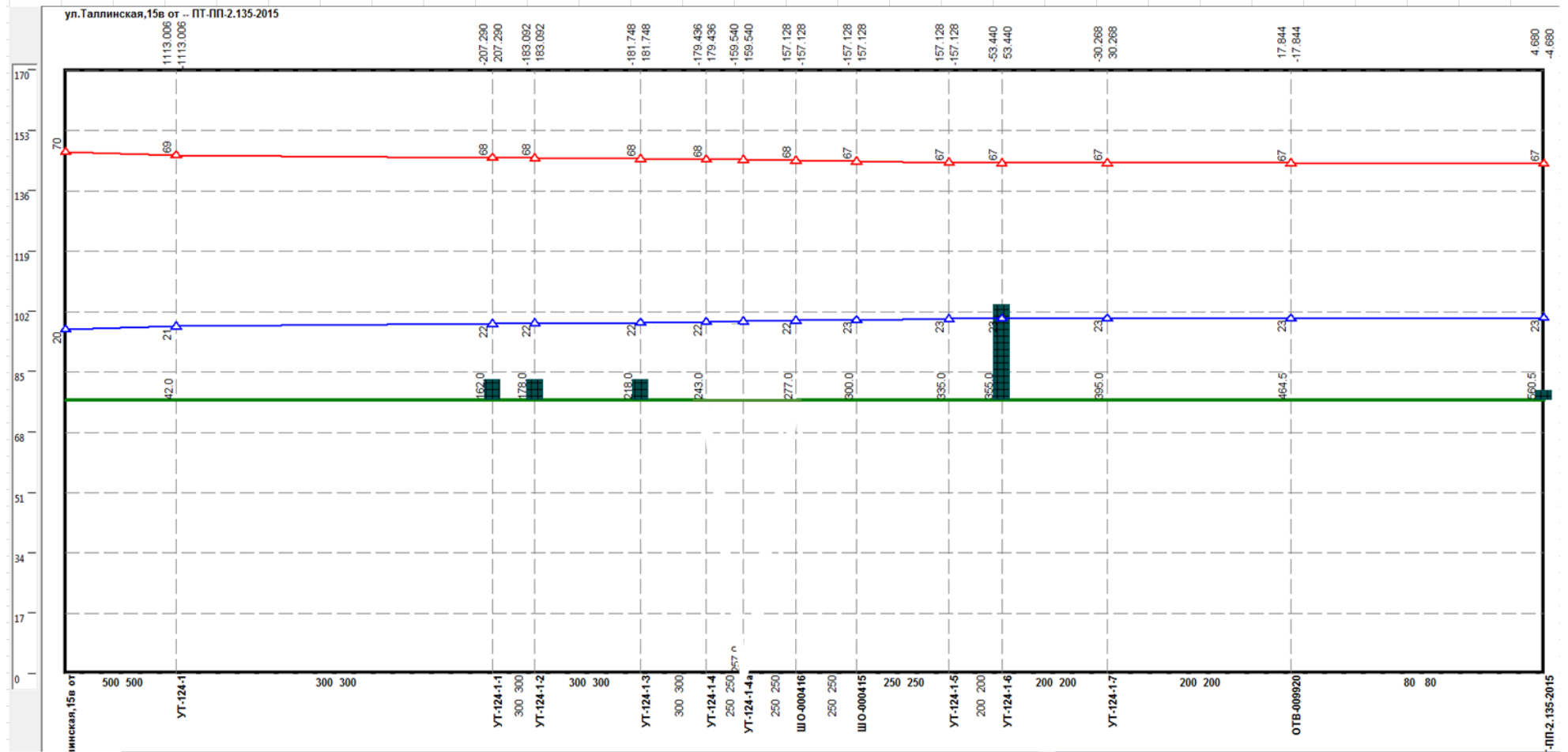
Рисунок 1.124 –Результат гидравлического расчета - график гидравлических режимов по пути теплоносителя от котельной Таллиннская, 15в до ОТВ-009920
