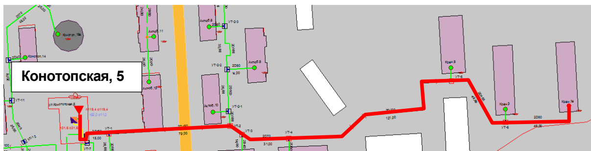
Рисунок 1.95 – Результат гидравлического расчета - расчетный путь теплоносителя от котельной Конотопская, 5 до ПТ-Кран,1а
