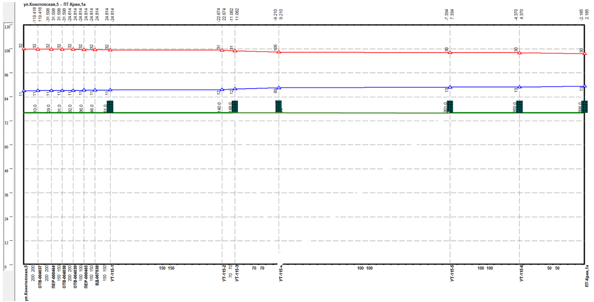
Рисунок 1.96 –Результат гидравлического расчета - график гидравлических режимов по пути теплоносителя от котельной Конотопская, 5 до ПТ-Кран, 1а
